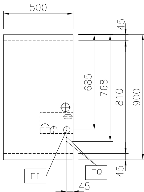
Boven aanzicht
